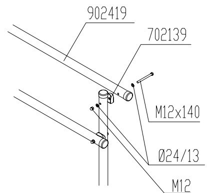
DET 3
